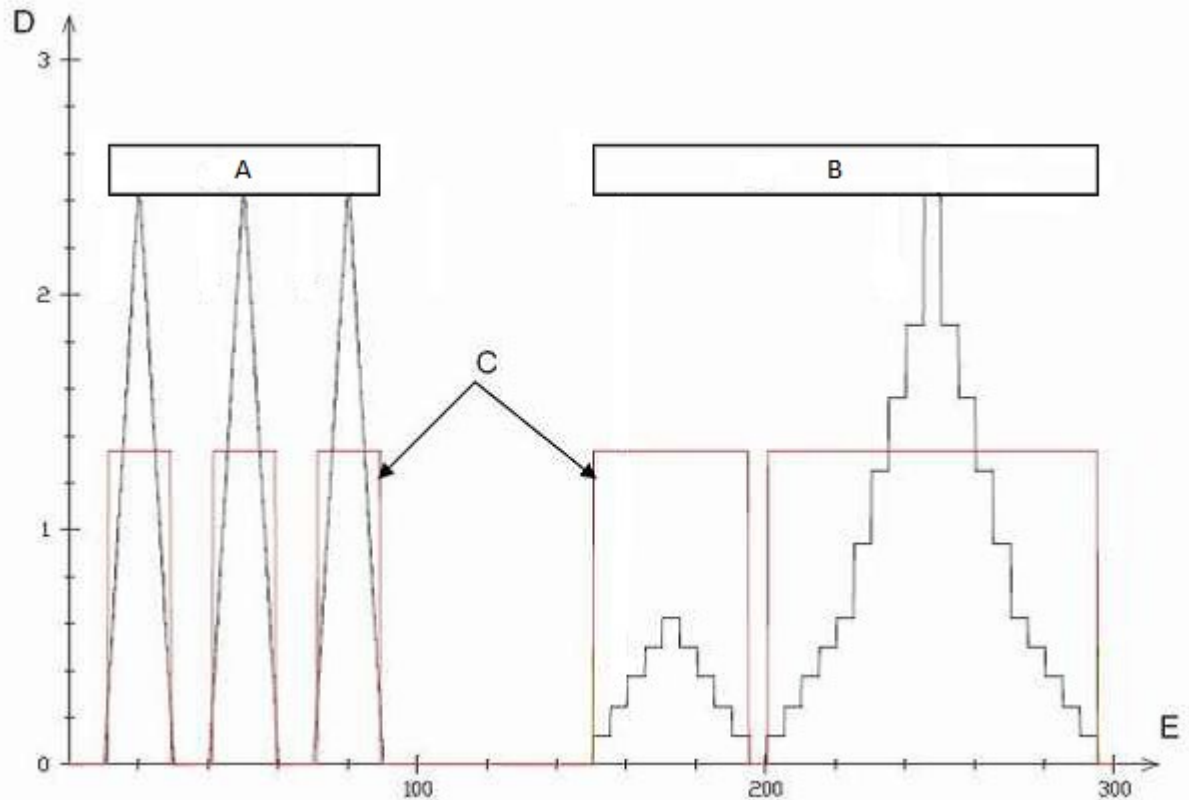
Figure 7 : Cycle électrique
